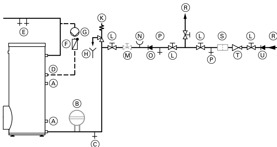
Abb. 15 Beispiel: 300 l Inhalt
